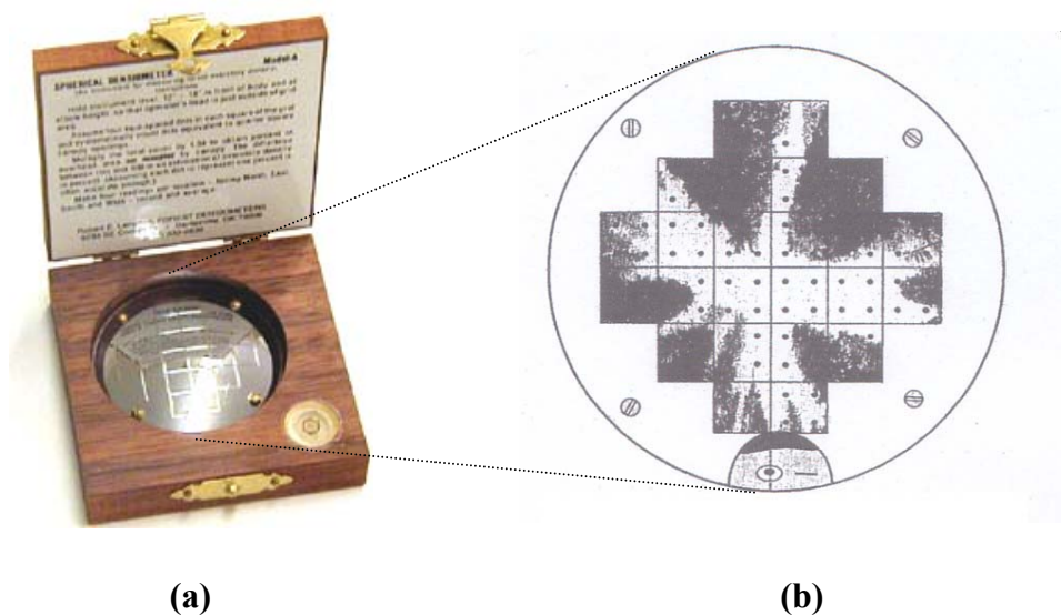
Figura 7. Densiômetro esférico côncavo (a) e a representação visual da sua utilização no campo (b) para determinação da abertura do dossel (área não escurecida pela vegetação) nas parcelas experimentais da UT 14, UPA 7, Fazenda Rio Capim, Paragominas-PA.
